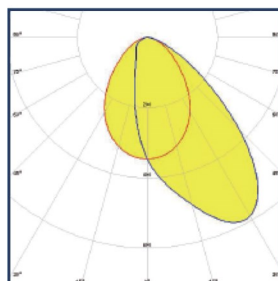
Lentille asymétrique
